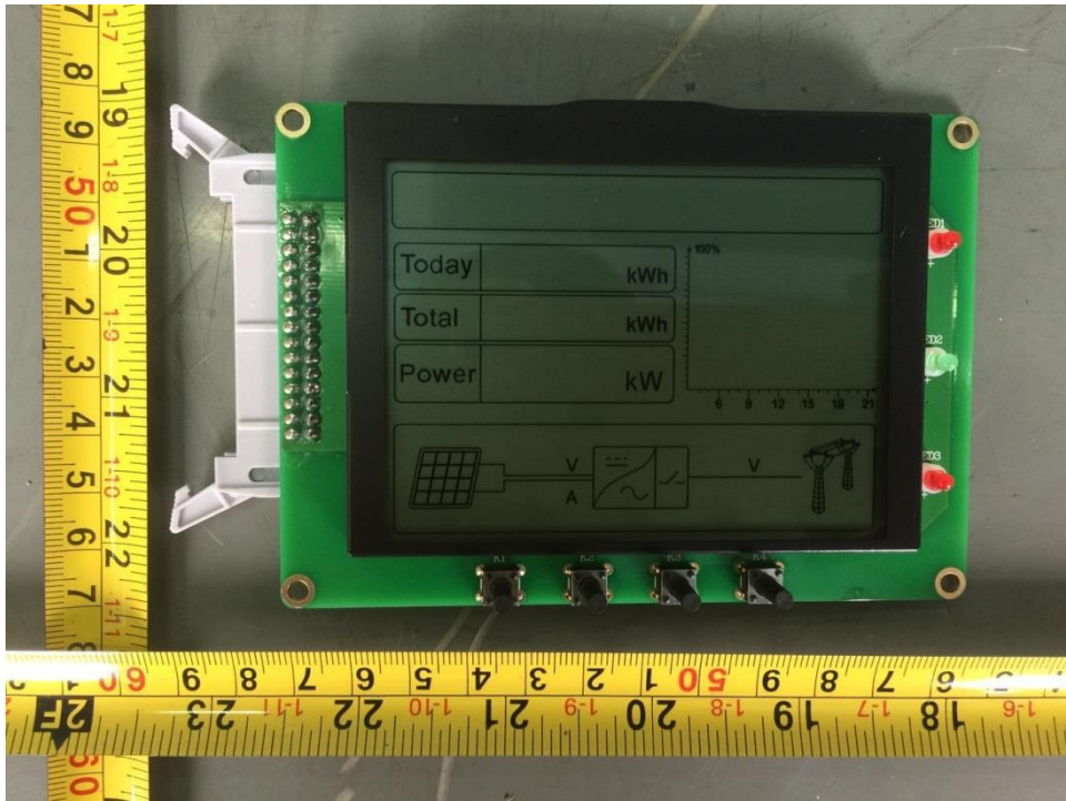
图 6 LCD 板正面
