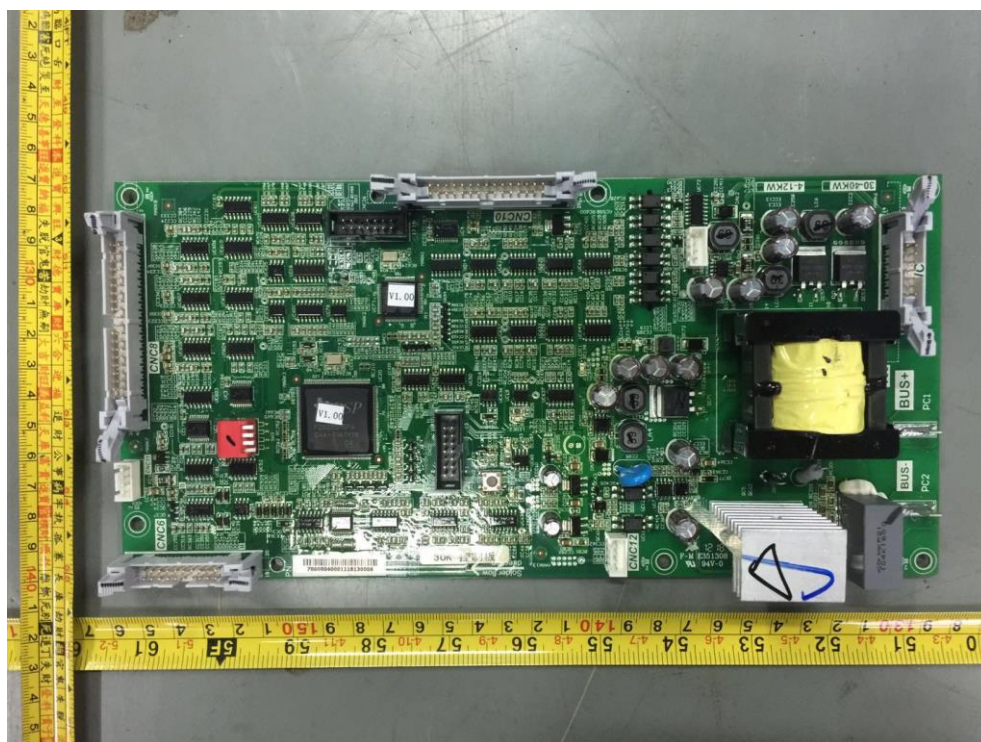
图 8 控制板正面
