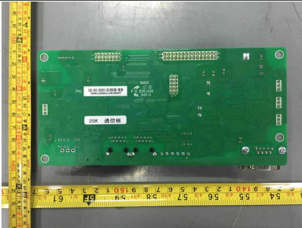
图 15 通讯板背面
