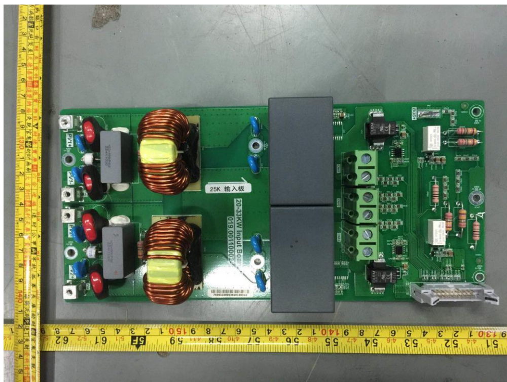
图 12 输入板正面
