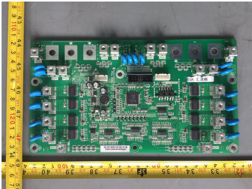
图 16 汇流板正面
