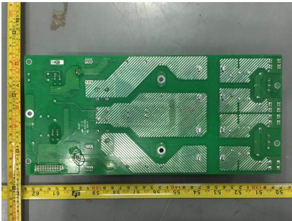
图 13 输入板背面
