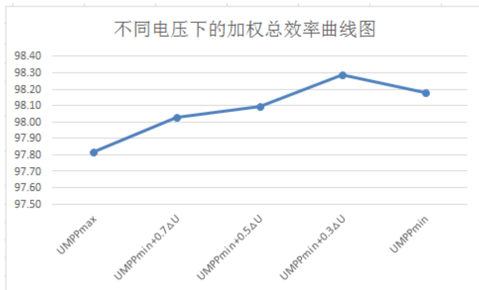
模拟晶硅组件的不同电压下的加权总效率曲线
