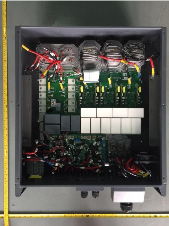
图 3 内部结构
