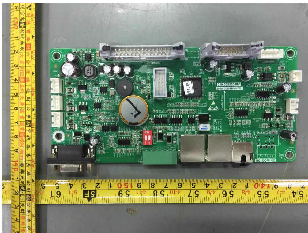
图 14 通讯板正面
