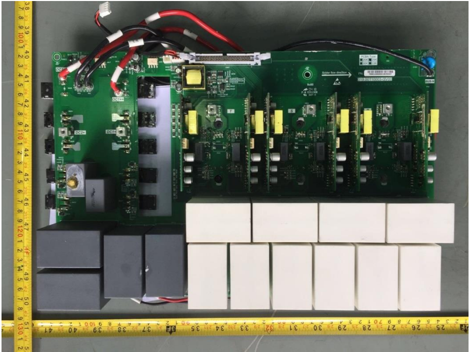
图 4 主板正面
